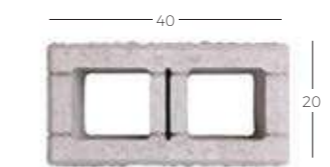
Pustak podmurówkowy - rozszczepiany z dwóch stron
