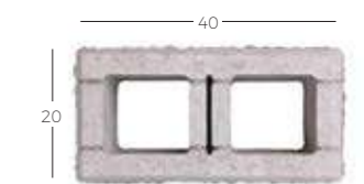
Pustak słupkowy - rozszczepiany z czterech stron
