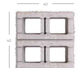
Pustak podwójny - rozszczepiany z czterech stron
